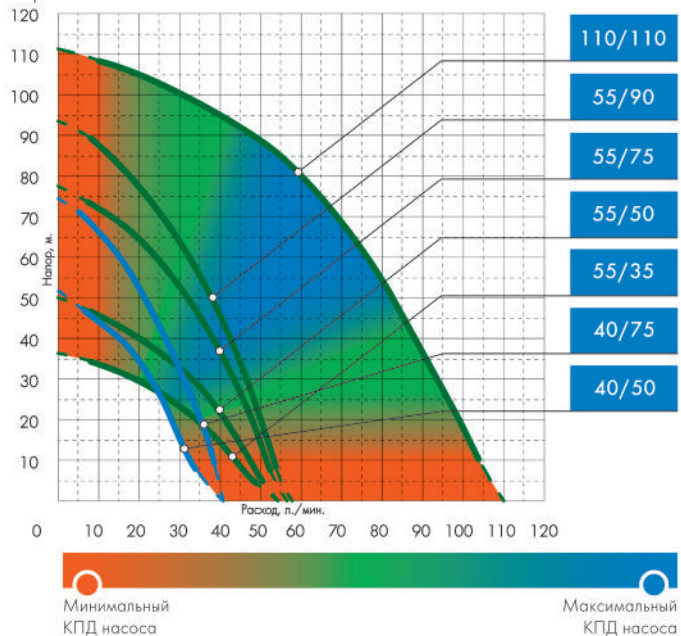
График напорных характеристик*:
